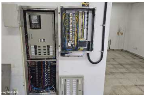
안록역 원격조명제어용 제어반
